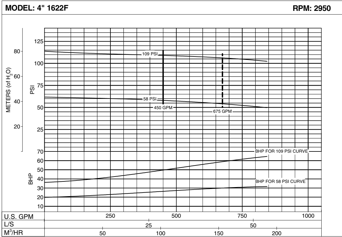
Curve No: PC-219399
