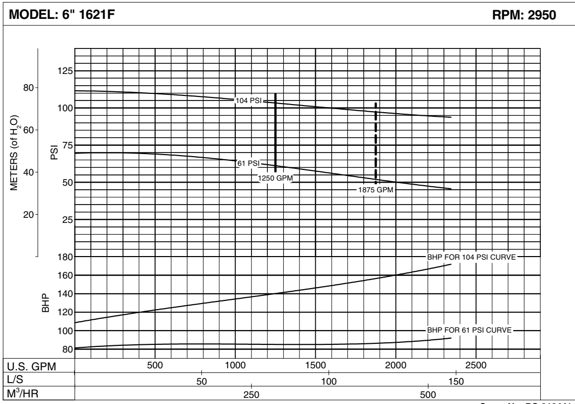
Curve No: PC-219441
