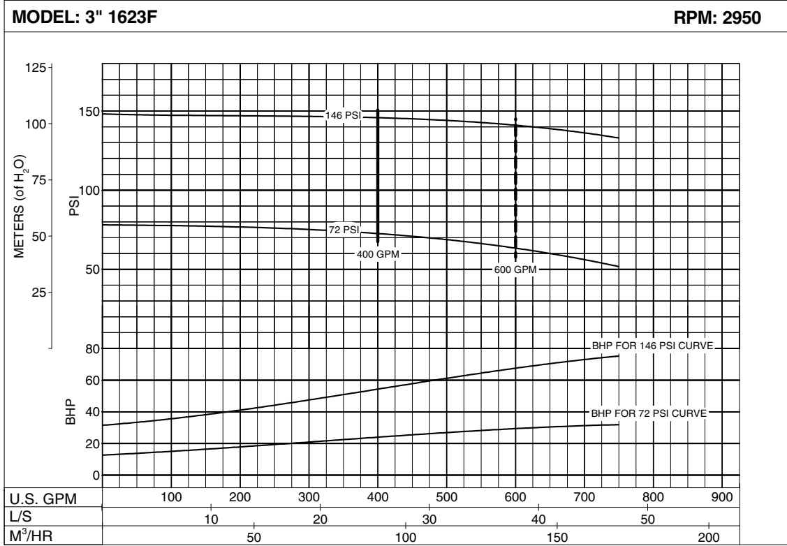
Curve No: PC-219291
