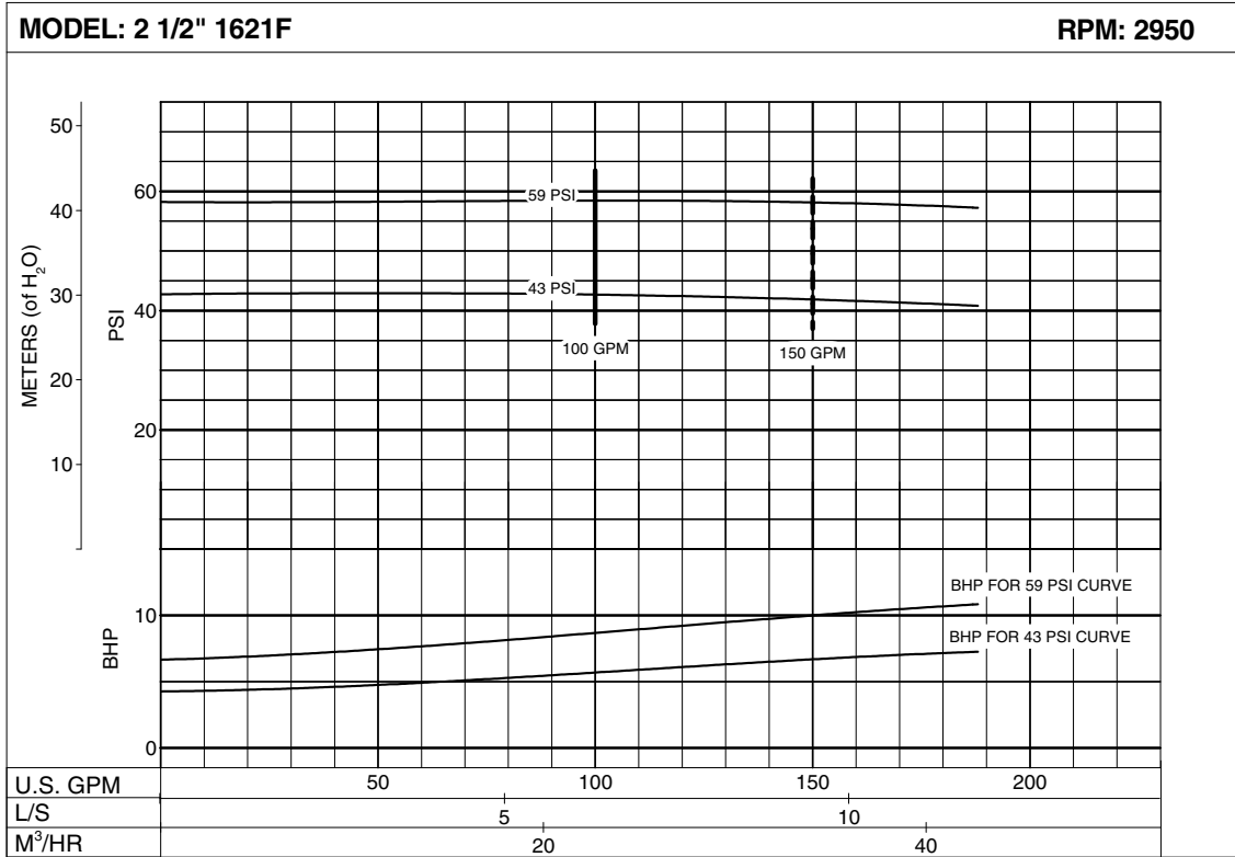
Curve No: PC-219204
