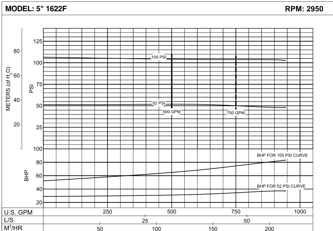
Curve No: PC-214666
