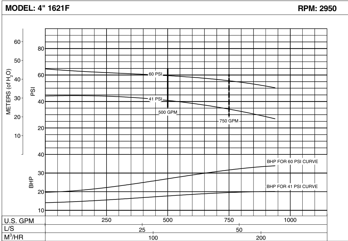
Curve No: PC-219357
