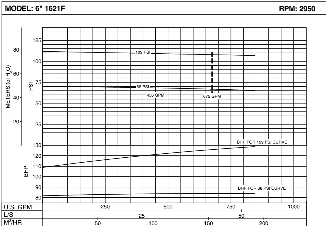
Curve No: PC-219437
