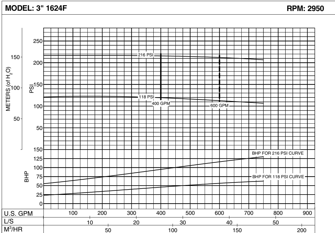
Curve No: PC-219341
