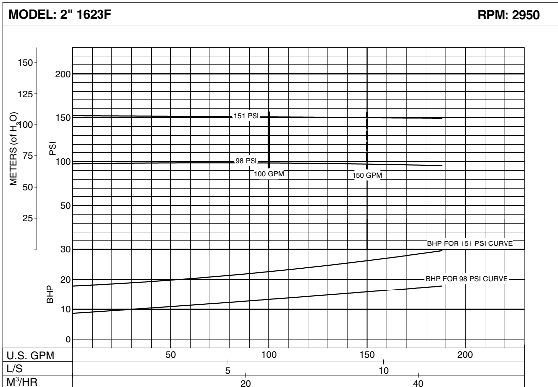
Curve No: PC-219244
